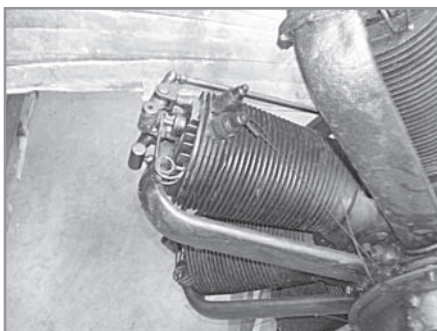
Глава цилиндра; види се издувни вентил и две свећице
