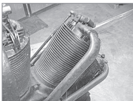
Глава цилиндра; види се улисни вентил и цев за сировод мешавине горива и ваздух
