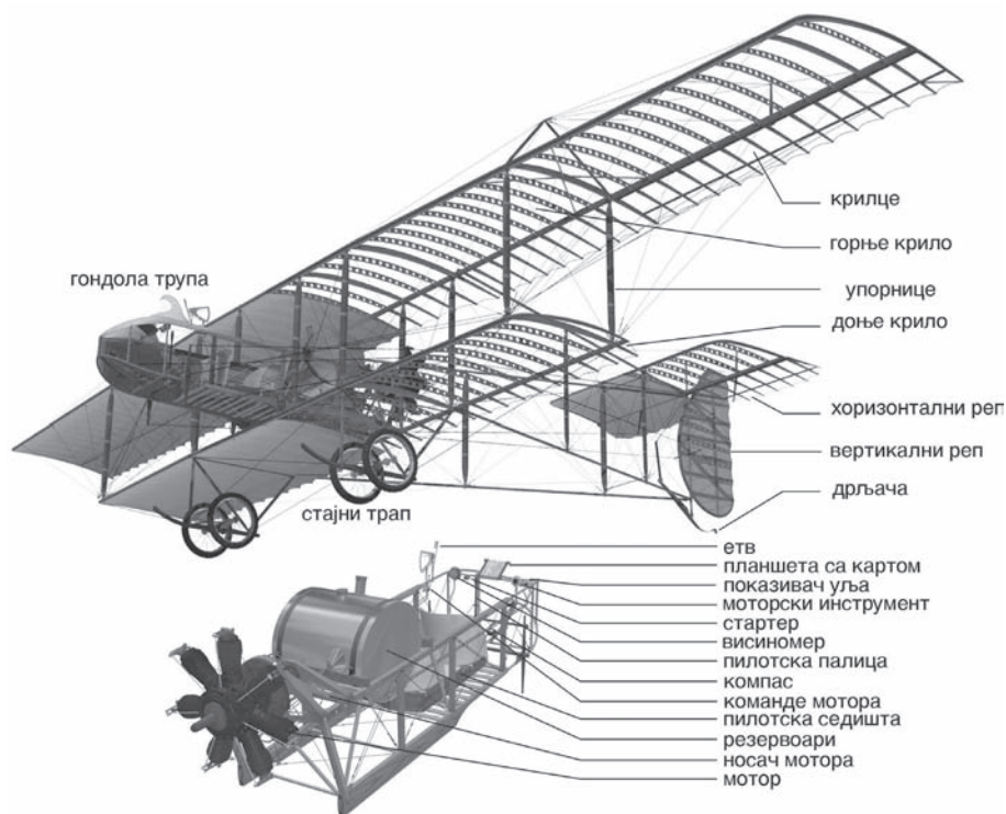
Конструкција и кабина Француској авиона Анри Фарман HF 20. Представља класичну конструкцију раног доба авијације
