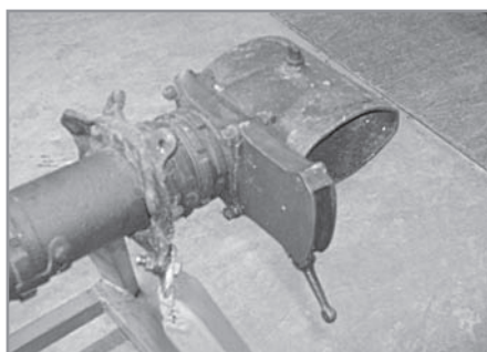
Детаљ уписа карбуратора, полуће регулатора проточа ваздуха и задњеј окова за везу са шрумом
