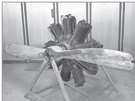
Музејски примерак мотора Клерже 9Б5 у дейоу
